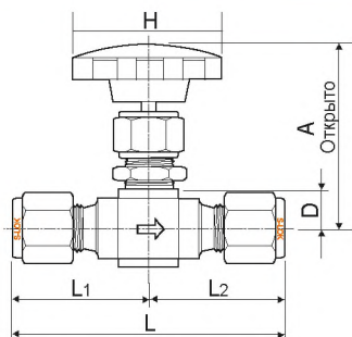
Прямой
