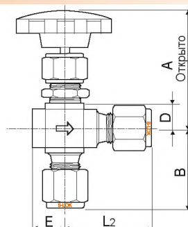
Угловой
